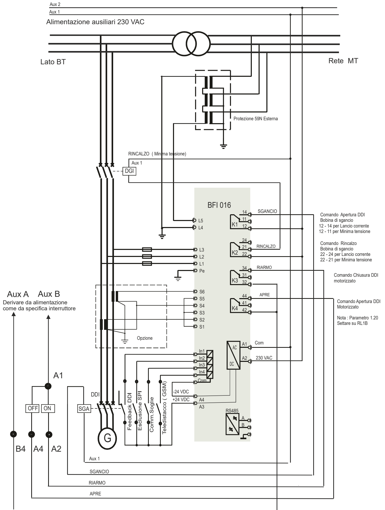
BFI 16 Schema di installazione di principio DDI Interruttore Motorizzato
